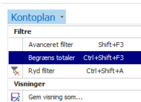
Figur 11 – Begræns totaler
